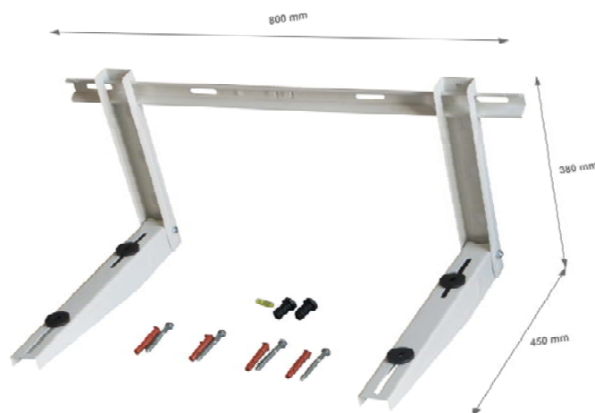
Skladacia konzola BA - Set vrátane hmoždín skrutiek vodováhy antivibračných podložiek rozмеры 800x380x450mm cena 9,9 Eur/pár
